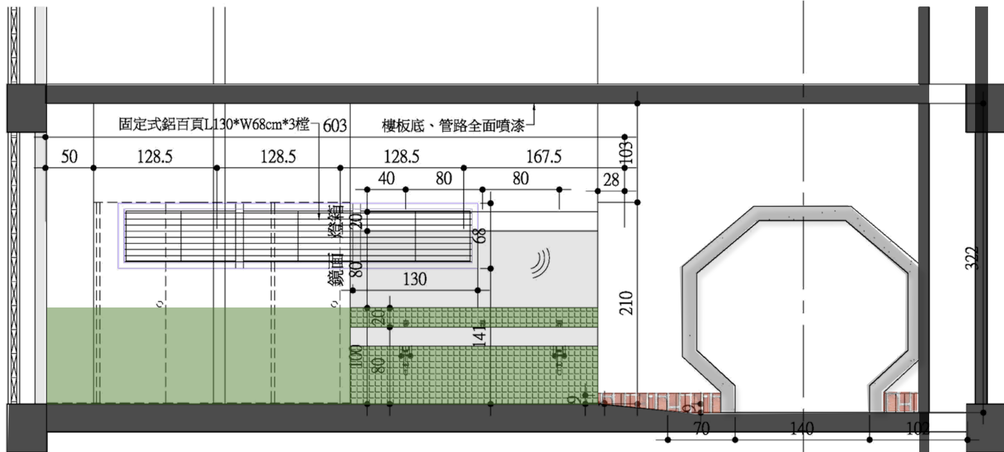
1F北向剖立面圖(改善後) (松軒)
