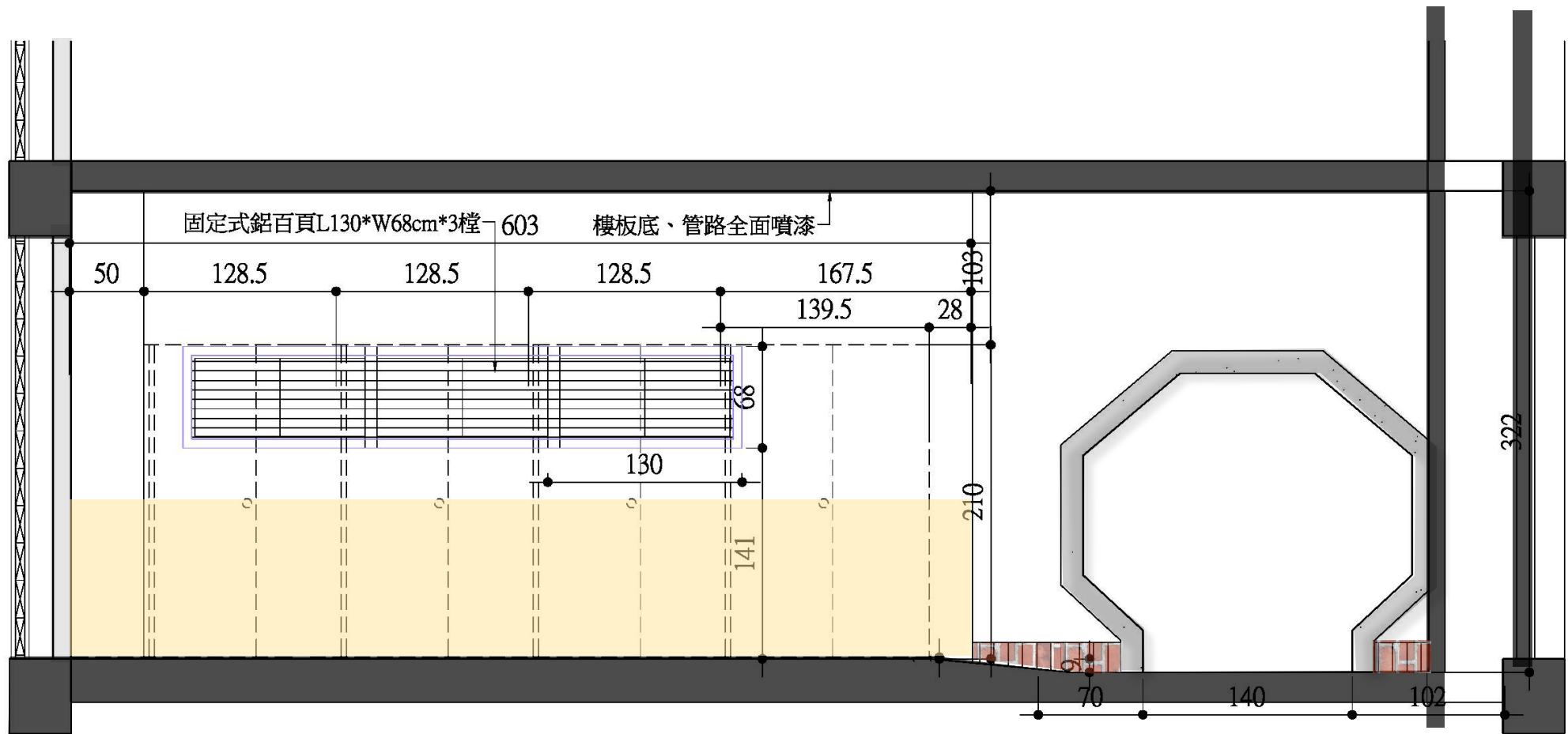
5F北向剖立面圖(改善後) (菊軒)
