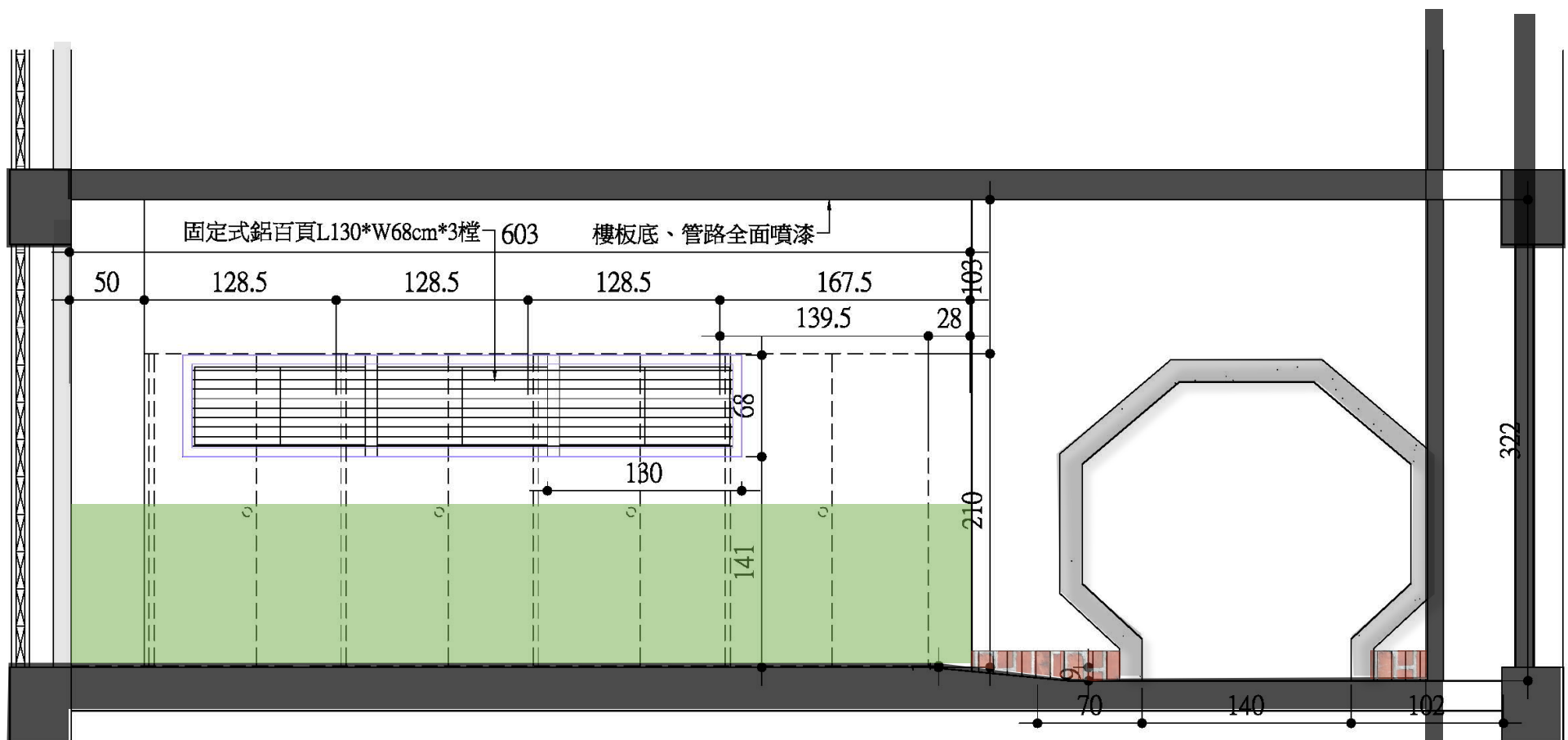
2F北向剖立面圖(改善後) (竹軒)
