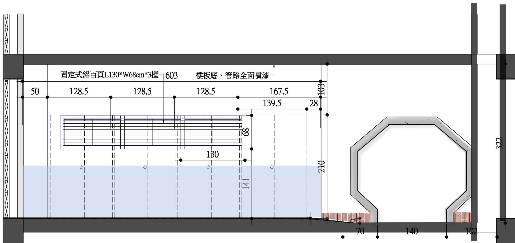
4F北向剖立面圖(改善後) (蘭軒)
