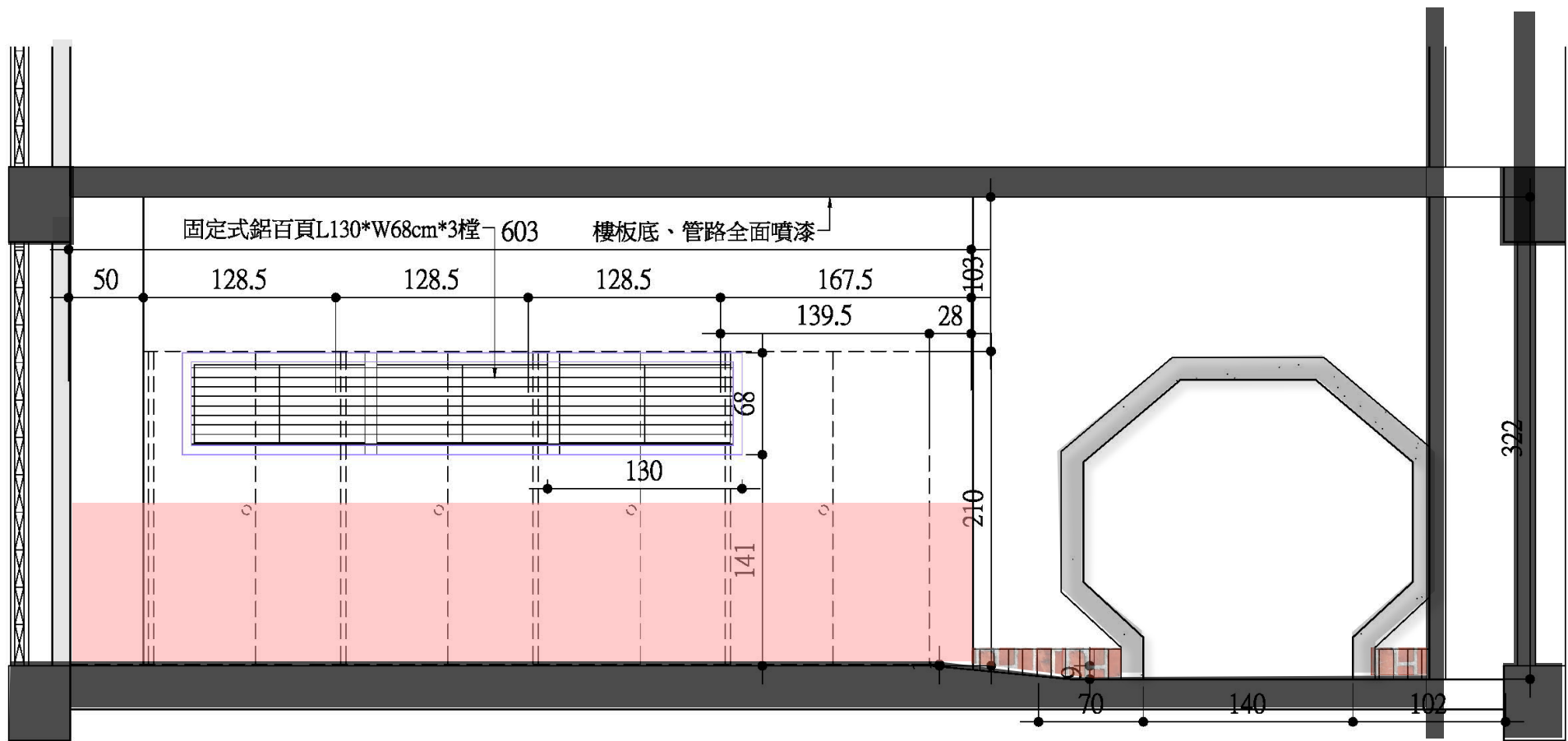
3F北向剖立面圖(改善後) (梅軒)
